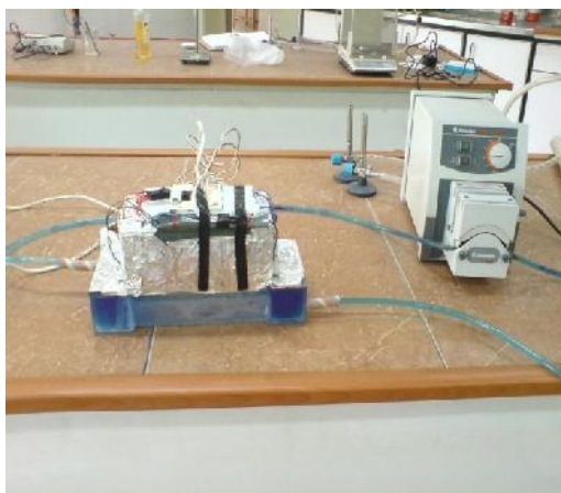
شکل ۲- راکتور متصل به پمپ پریستالتیک
