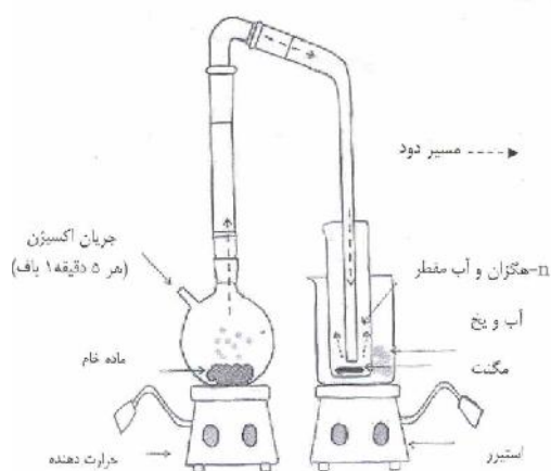
شکل ۱. شمایی از دستگاه طراحی شده و نحوه تولید و جمع آوری دود دارویی عنبر نسارا مطالعات بیولوژیک
