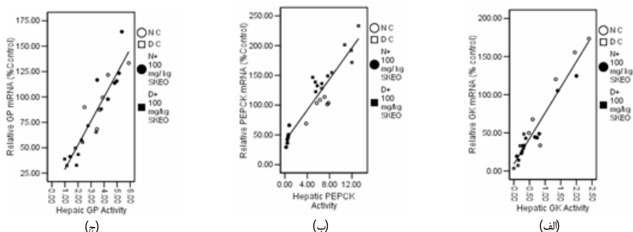
شکل شماره 3- همبستگی بین سطوح mRNA و فعالیت‌های یک آنزیم خاص. میزان همبستگی ها: الف - با r=0/961 برای GK، ب - با r=0/931 برای PEPCK و ج - با r=0/926 برای GP در p < 0/01 معنی دار است. اعداد بکار رفته جهت رسم این نمودار بترتیب با اعداد قبلی فعالیت (شکل 1) و سطوح mRNA (شکل 2) برای یک آنزیم خاص یکسان است.
