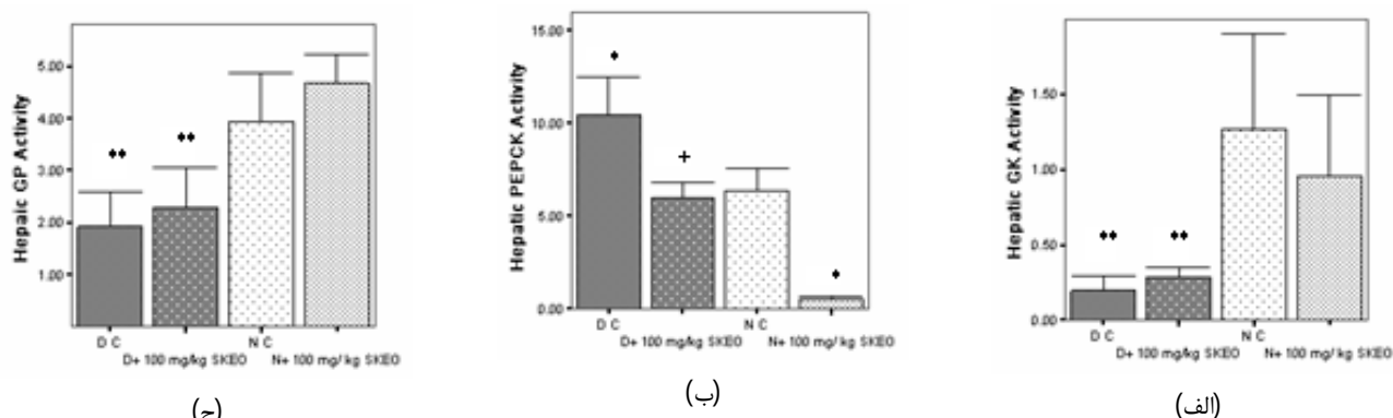
شکل شماره 1- اثر تجویز SKEO نوع بومی بر فعالیت آنزیم‌های کبدی: الف- GK، ب- PEPCK، ج- GP. نرمال (N)، کنترل نرمال (NC)، دیابتی (D) و کنترل دیابتی (DC). مقادیر (means ± S.E. M) از هر گروه دارای 6 رت بدست آمد. 1. p < 0/05 و 2. p < 0/01 در قیاس با گروه کنترل نرمال و 3. p < 0/001 در قیاس با گروه کنترل دیابتی بدست آمده است. فعالیت آنزیم بصورت نانومول بر میلی گرم پروتئین در دقیقه محاسبه شده است.
